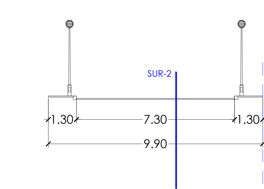
SECCIÓN Calle del Río Ebro (Existente)
