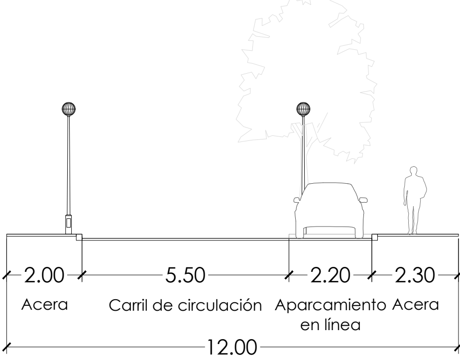
SECCIÓN (12 m) Viales 1,2,6,7, 8 y 10
