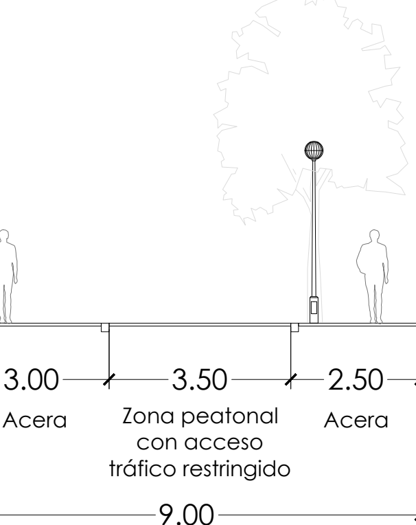
SECCIÓN (9 m) Vial 3
