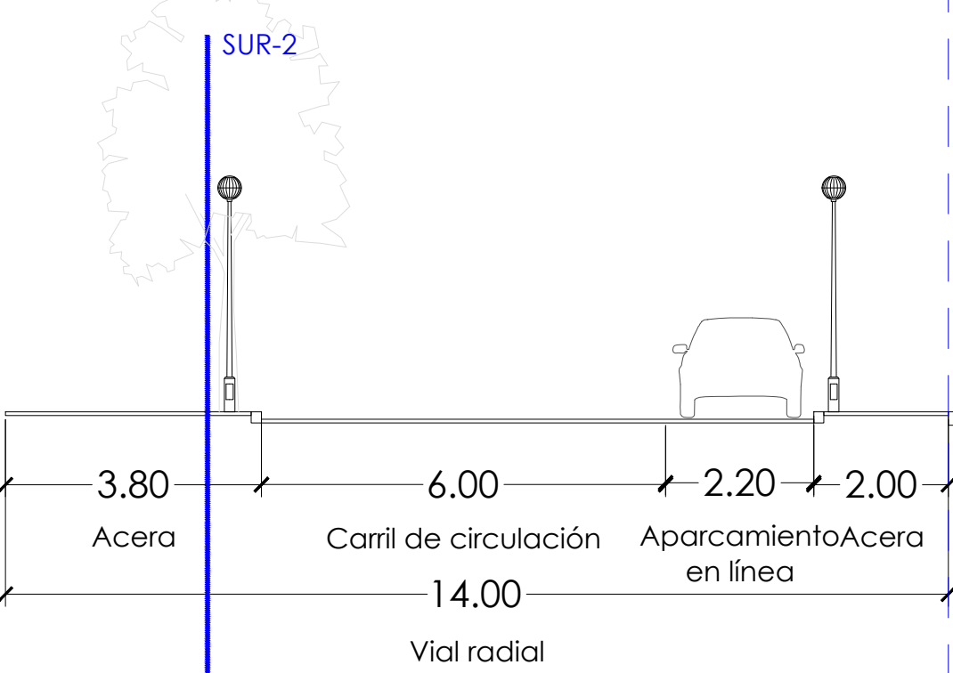
Sección Vial-Radial (14 m) continuación Calle Miguel Hernández
