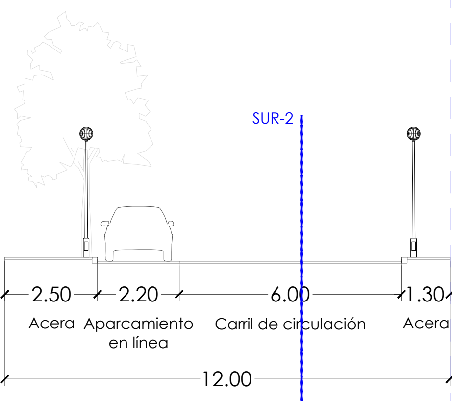
Sección Calle del Río Ebro (12 m) Vial 5
