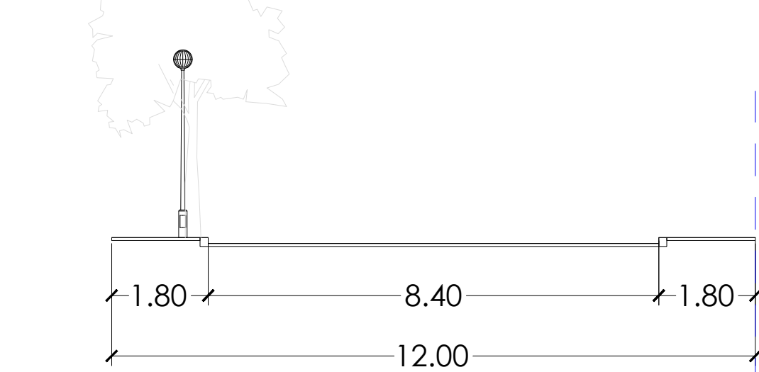
SECCIÓN Calle Miguel Hernández (existente)
