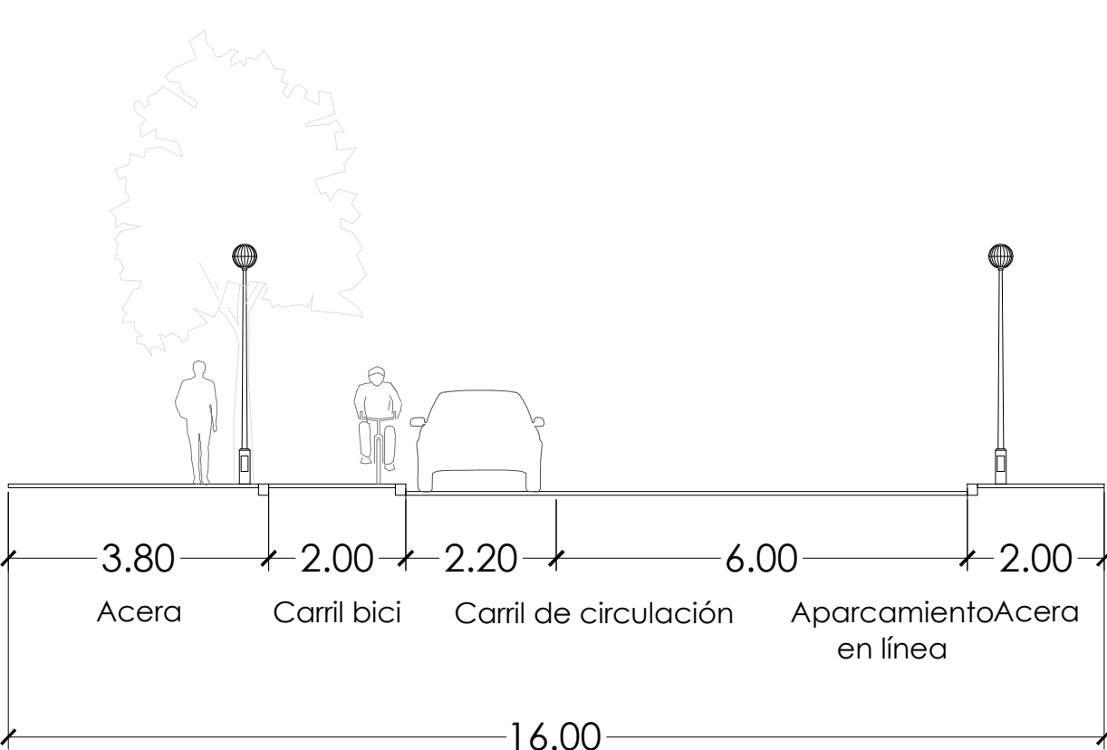
SECCIÓN Vial Perimetral (16 m)
