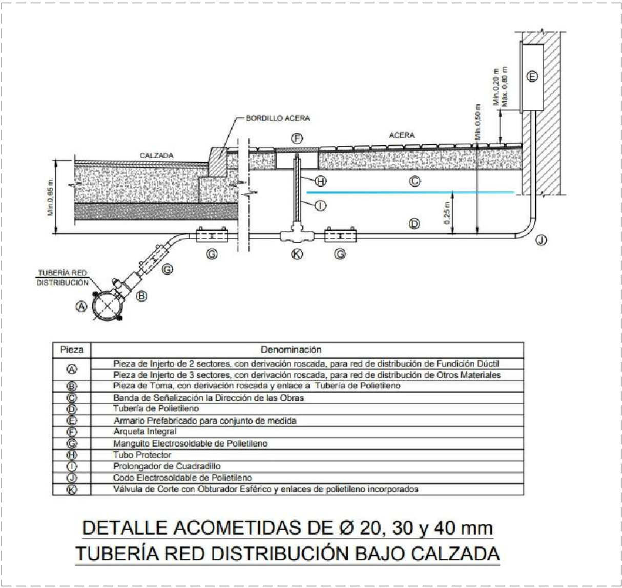
ACOMETIDA. SECCIÓN CONSTRUCTIVA
