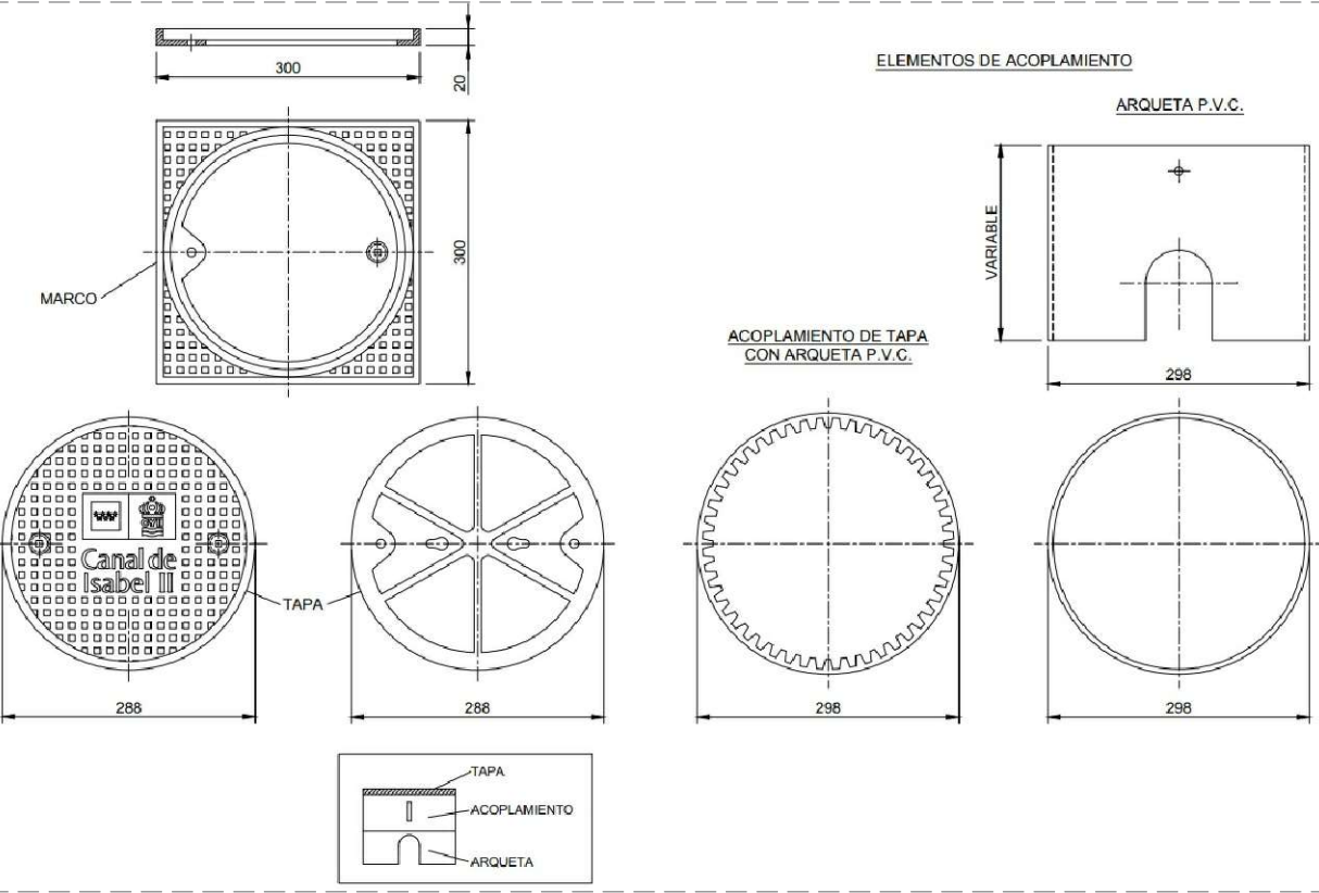
ARQUETA INTEGRAL ACERA
